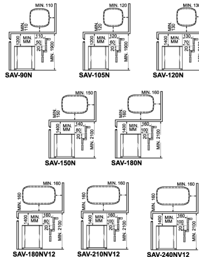
Fig. 2 Рис. 2 Distances minimales de sécurité Минимальное безопасное расстояние (мм)
