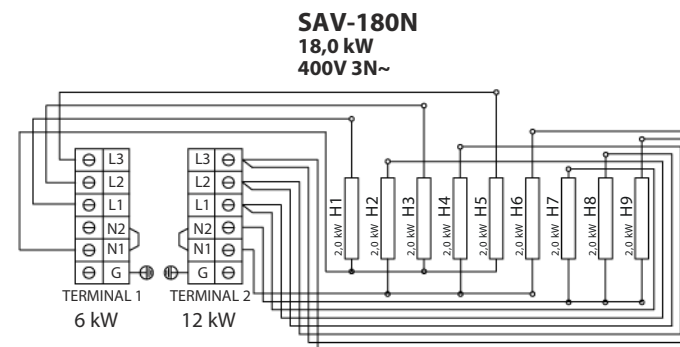
Fig. 6 Рис. 6 Eléments de chauffage Элементы нагрева
